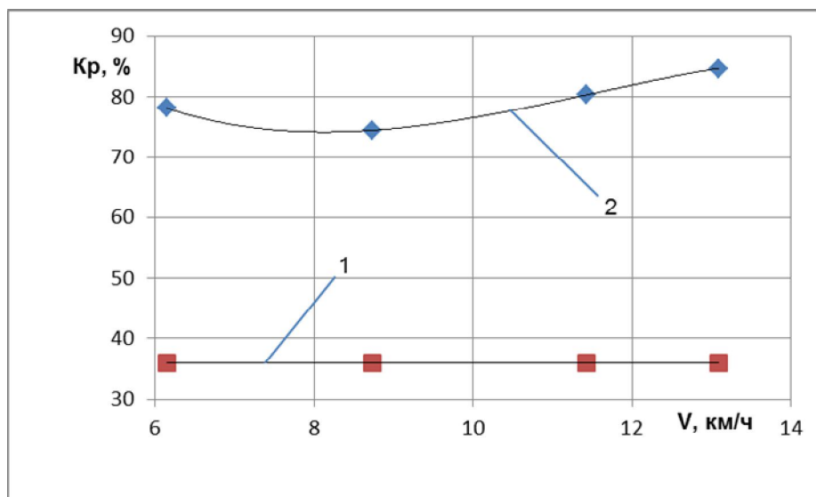
Рисунок 3 - Зависимость крошения почвы от скорости движения:
