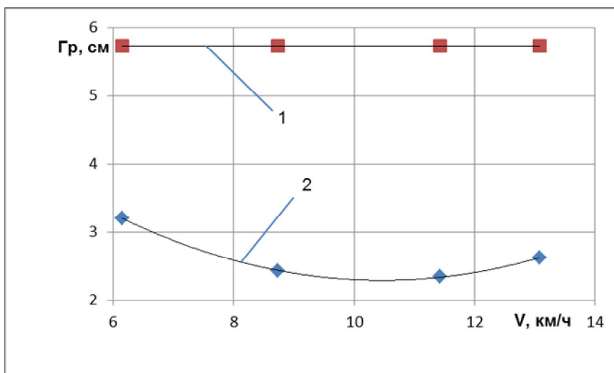
Рисунок 2 - Зависимость гребнистости поверхности поля от скорости движения:
