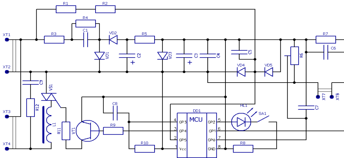
Рисунок 1- Принципиальная электрическая схема устройства
