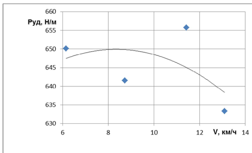
Рисунок 4 - Зависимость удельного тягового сопротивления орудия от скоростей движения
