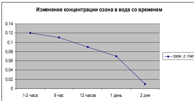
Рисунок 2 - Изменение концентрации озона в воде со временем
