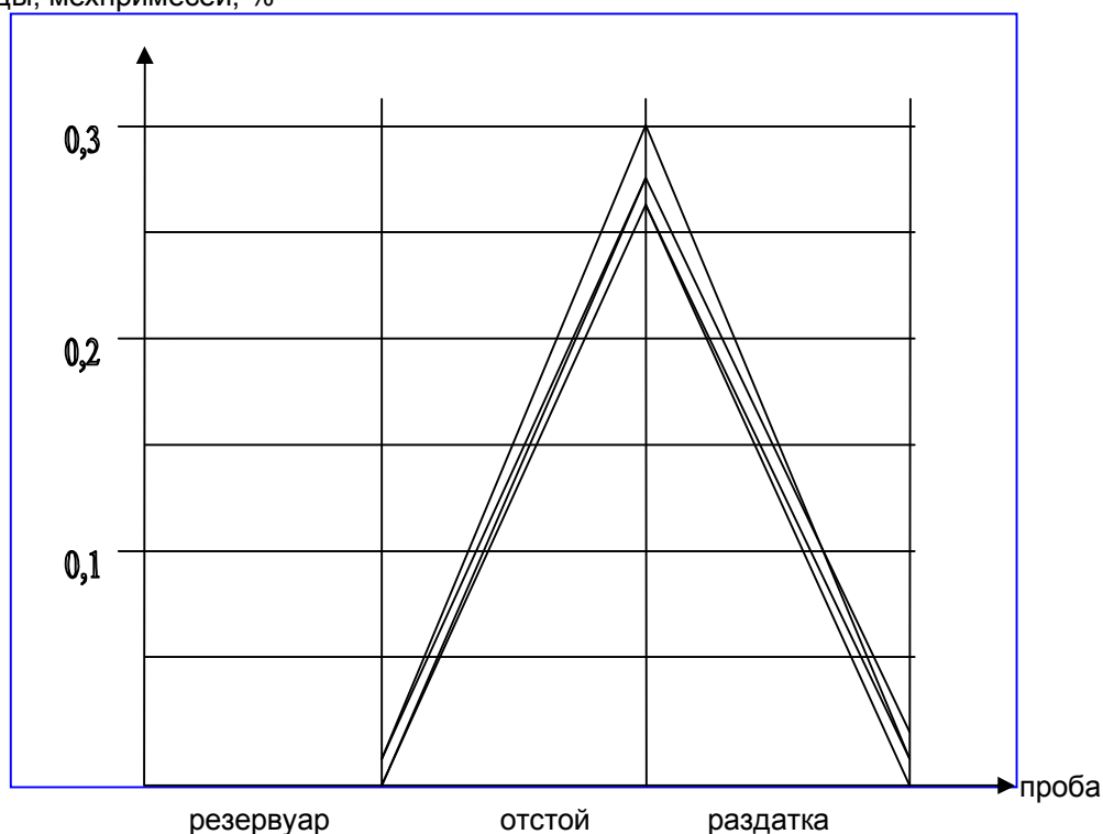
Рисунок 2 - Сравнительный график результатов исследований качества бензинов на наличие механических примесей и содержания воды
