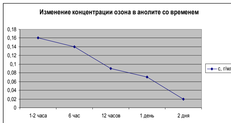
Рисунок 3 - Изменение концентрации озона в анолите со временем
