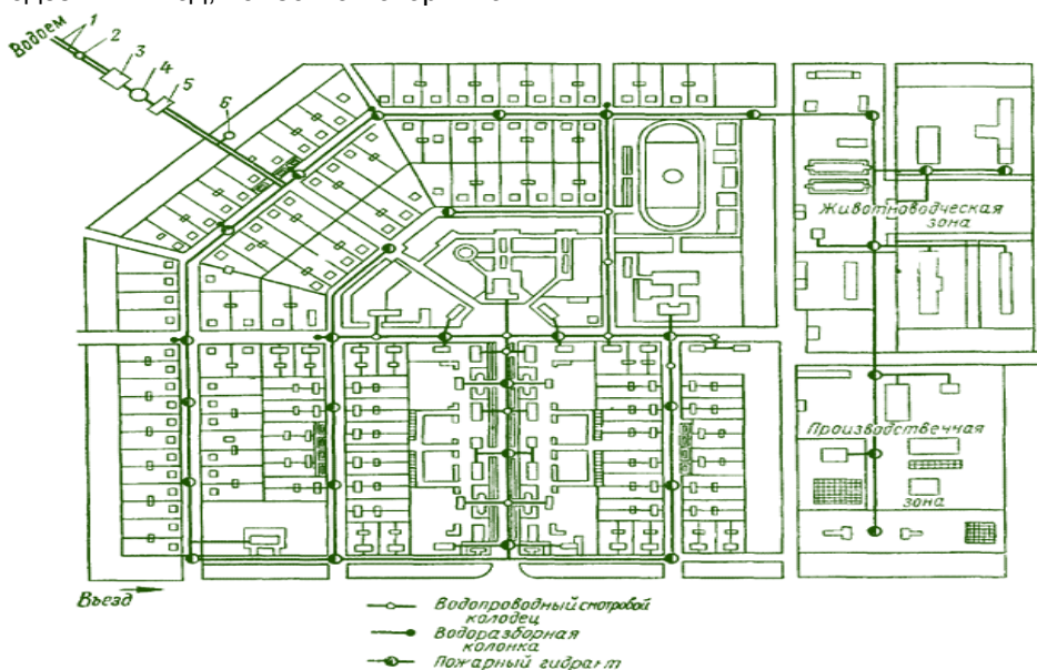
Рисунок 1 - Система водоснабжения центральной усадьбы хозяйства с использованием поверхностного источника
